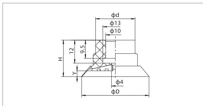
SFA35-50
